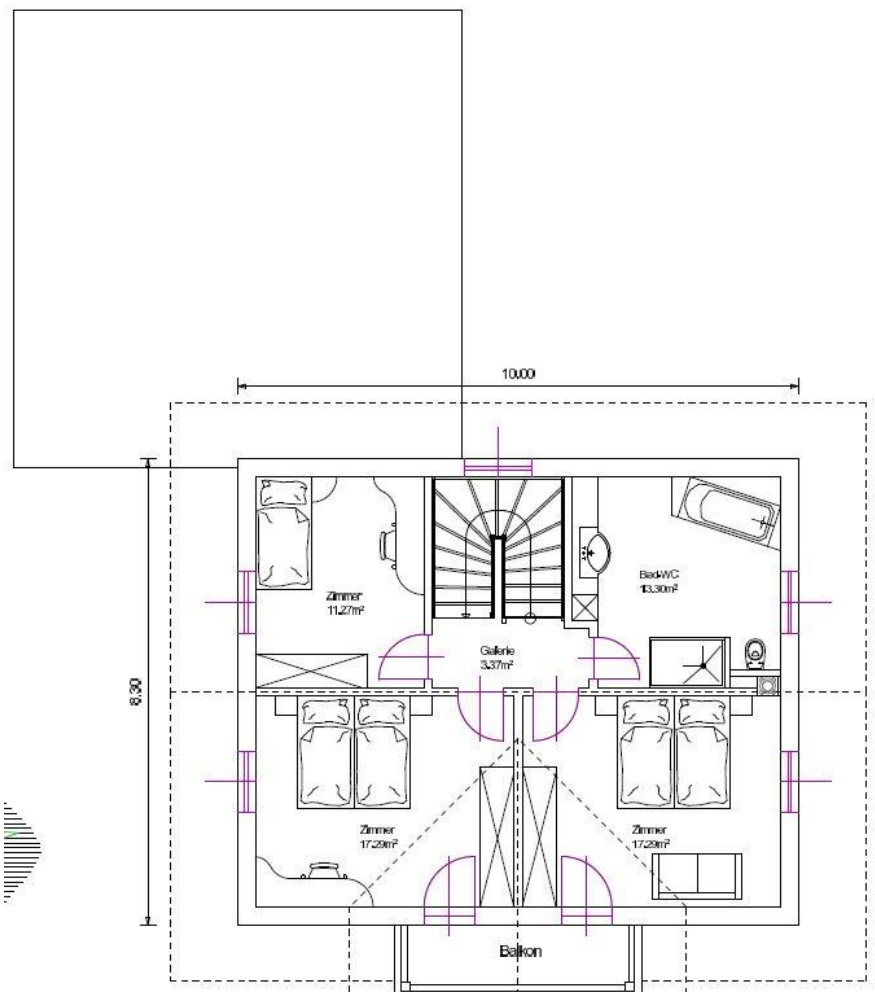
Grundriss Obergeschoss Wohnfläche Obergeschoss: ca. 62 m 2
